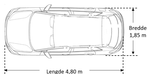
Figur 2.1: Dimensjonerende bil
