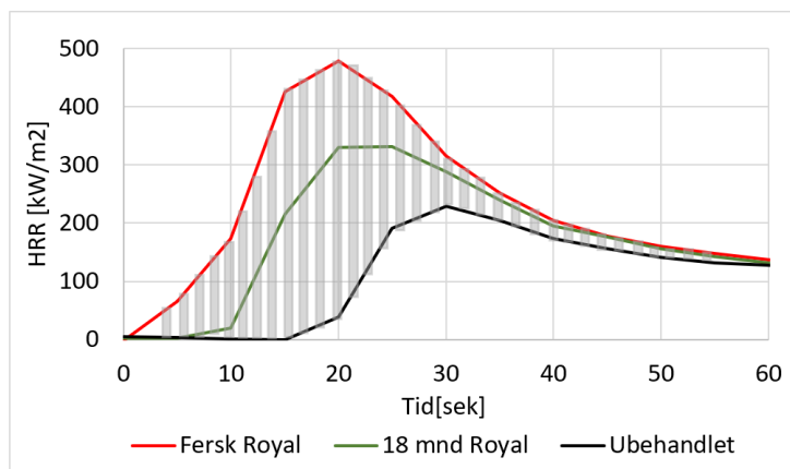
Figur nr. 4.2.: Varmeavgivelse (konkallorimeter) fra behandlet og ubehandlet kledning /7/
