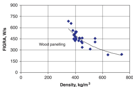
Figur 4-1 FIGRA-verdi for trepanel som funksjon av tetthet
