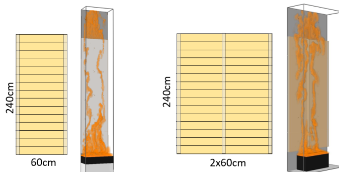
Figur nr. 6.4.: CFD modeller av liggende panel med henholdsvis et og to separate hulrom.
