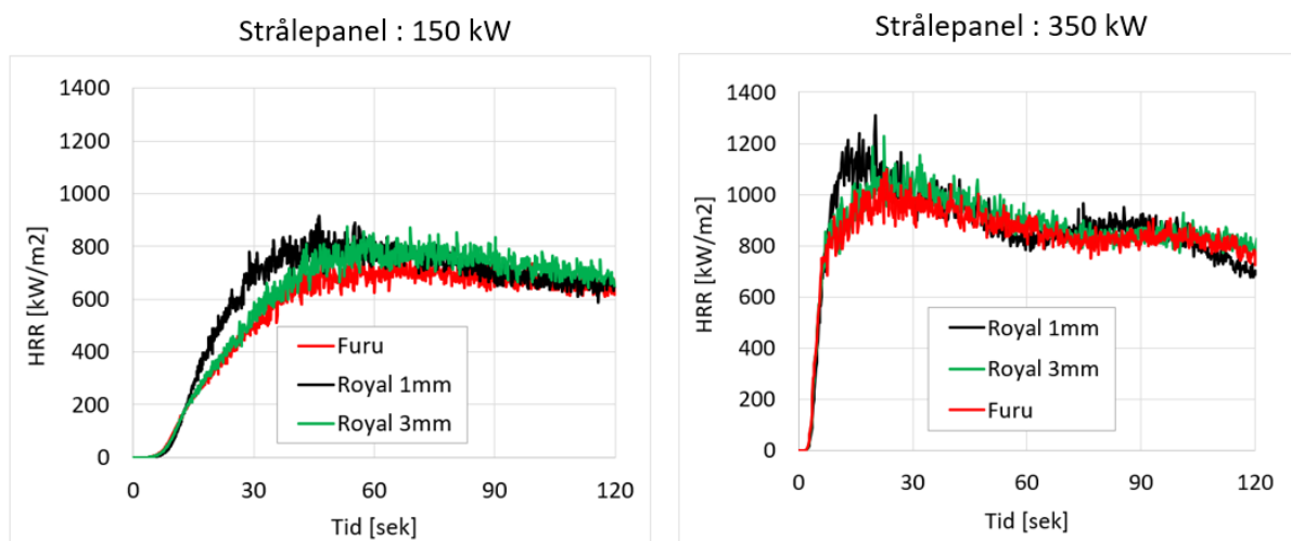
Figur 6-1 Varmeavgivelse fra utvendig panel som eksponeres fra strålepanel
