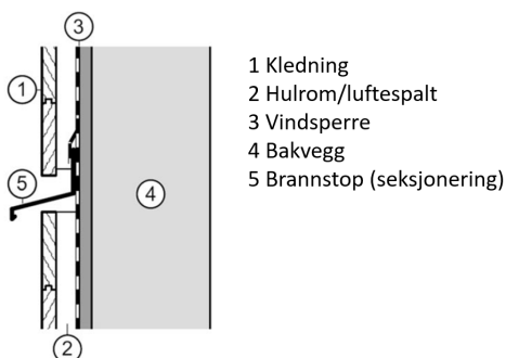
Figur nr. 3.2.: Vertikal seksjonering av kledning
